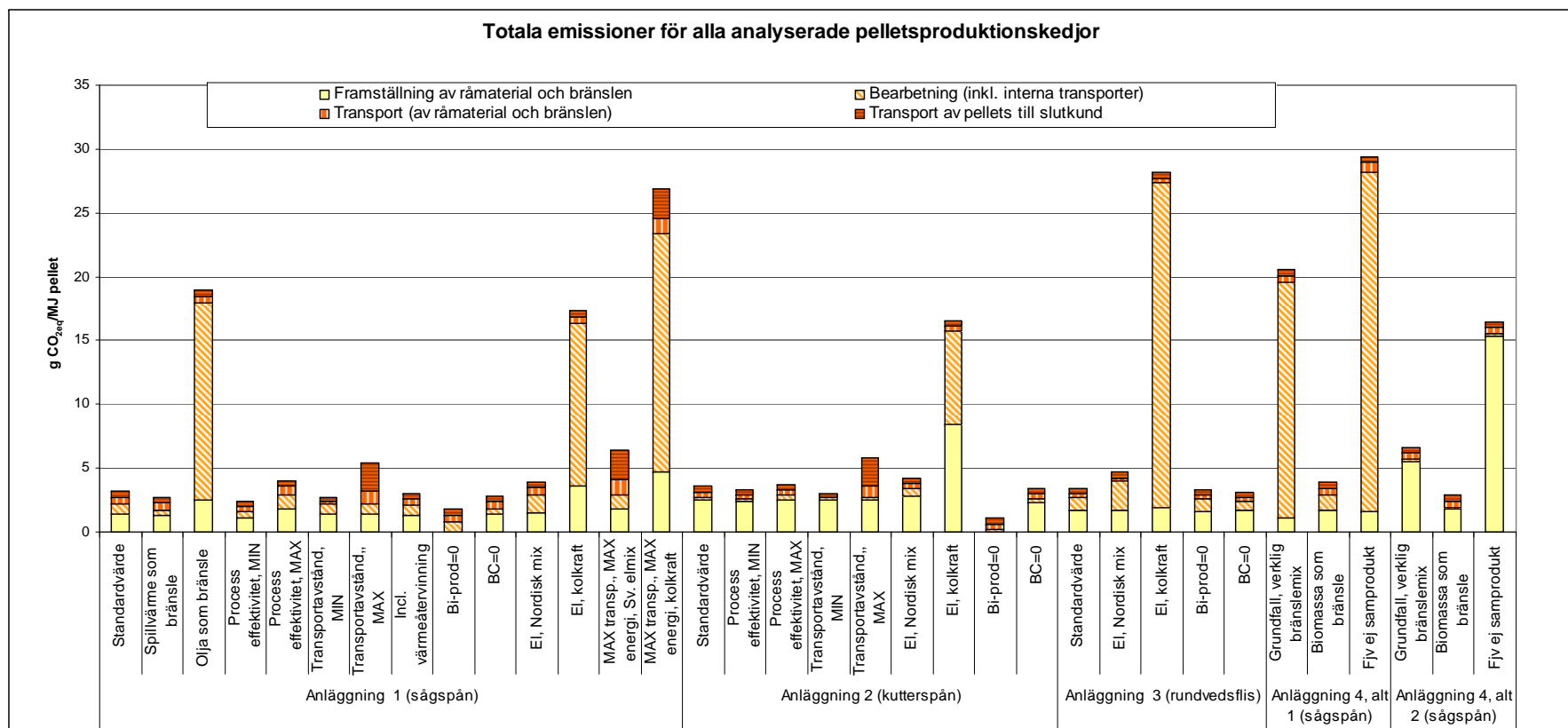
Figur S1 Sammanfattning av resultat för de olika analyserade pelletskedjorna. Anläggning 1-3 innebär produktion i fristående pelletsanläggningar. I Anläggning 4 sker produktion i pelletsanläggning integrerad med ett kraftvärmeverk (KVV) där alt 1) hela anläggningen betraktas som ett energikombinat och alt 2) pelletsanläggningen och KVV betraktas som separata anläggningar. Följande antagande används om inget annat anges: svensk elmix; typiska värden för processeffektivitet (energi) och transportavstånd; emissioner från produktion av biprodukter från sågverk och förbränning av biomassa medräknas; biomassa används för torkenergi i Anläggning 1 och 3; i Anläggning 4 antas verklig bränslemix i KVV (26% torv och 74% biomassa) och fjärrvärme betraktas som samprodukt. Förklaringar: Bi-prod=0 då emissioner från sågverksbiprodukter räknas till noll, BC=0 då alla förbränningsemissioner för biomassa räknas till noll, Fjv betyder fjärrvärme.
